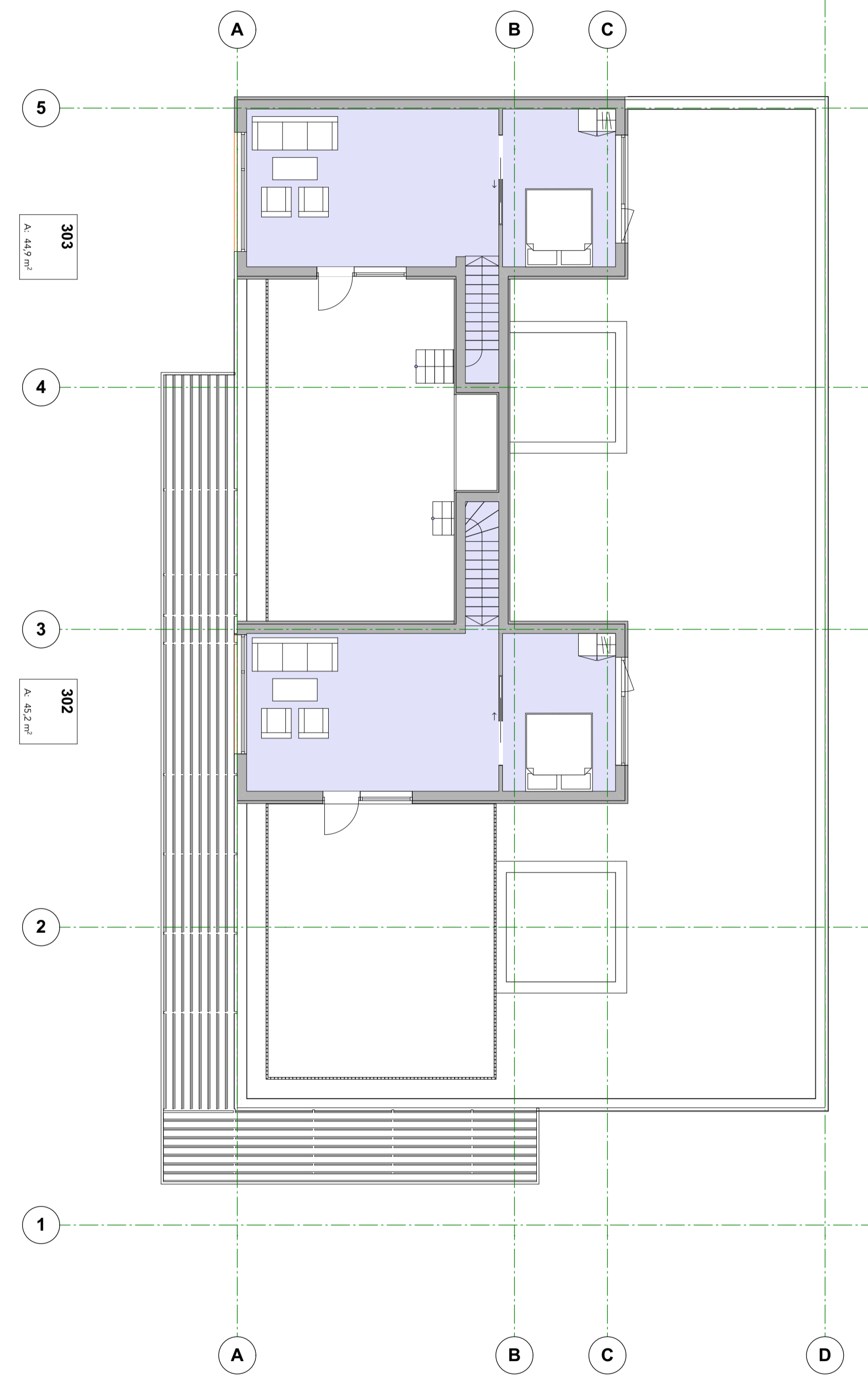
PLAN 3.ETG
