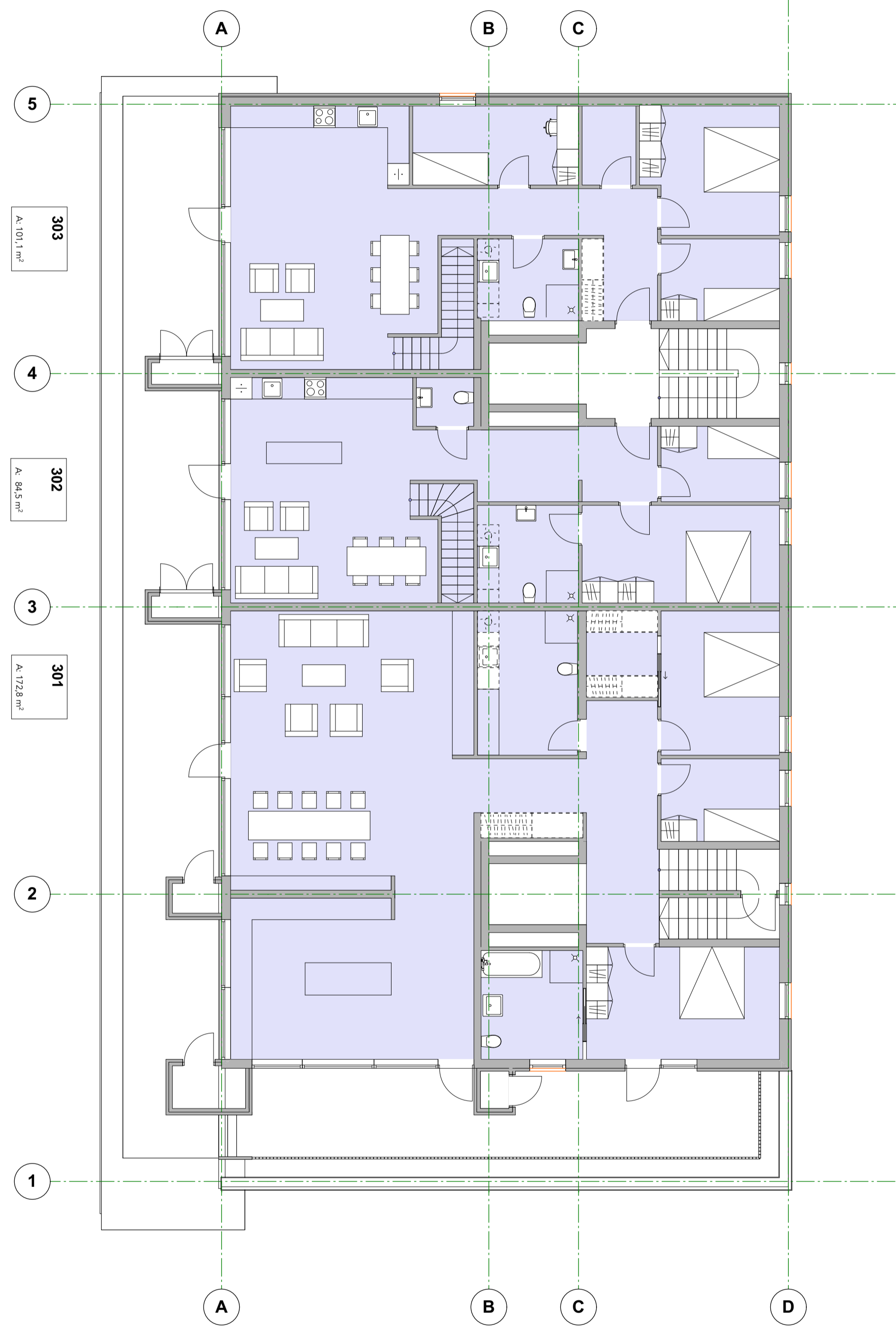
PLAN 2.ETG
